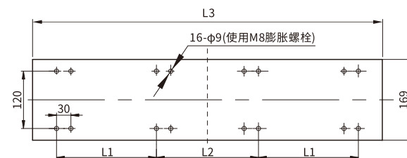
挂墙板尺寸
