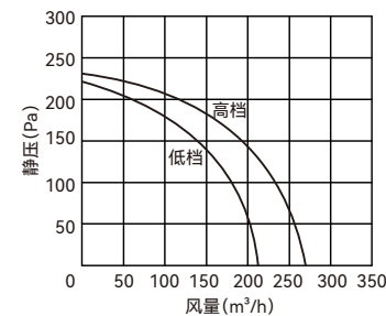
QFA-D250P(-Y) 静压-风量性能曲线
