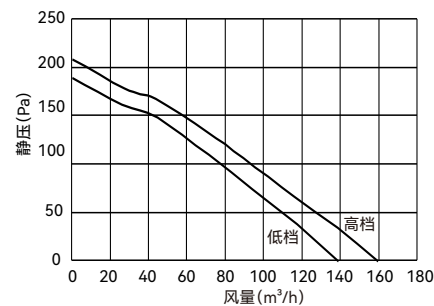
QFA-D150P(-Y) 静压-风量性能曲线
