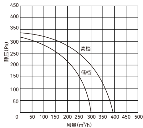
QFA-D350P(-Y) 静压-风量性能曲线
