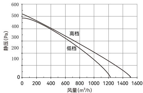
QFA-D1500P(-Y) 静压-风量性能曲线
