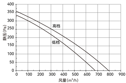
QFA-D800P(-Y) 静压-风量性能曲线
