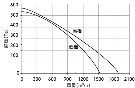
QFA-D2000P(-Y) 静压-风量性能曲线
