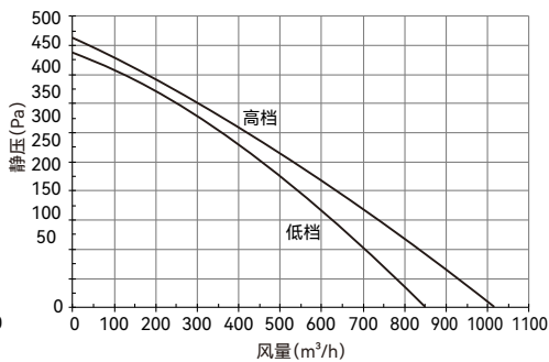
QFA-D1000P(-Y) 静压-风量性能曲线
