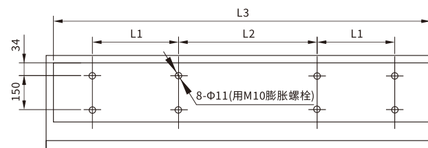
挂墙板尺寸图
