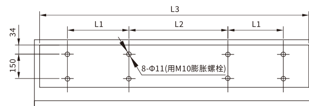
挂墙板尺寸图
