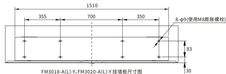
FM3018-A(L)-Y, FM3020-A(L)-Y 挂墙板尺寸图
