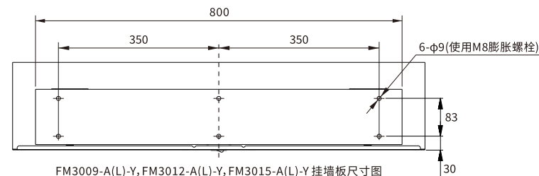
FM3009-A(L)-Y, FM3012-A(L)-Y, FM3015-A(L)-Y 挂墙板尺寸图
