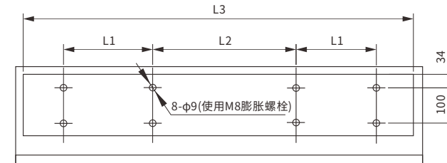
挂墙板尺寸图
