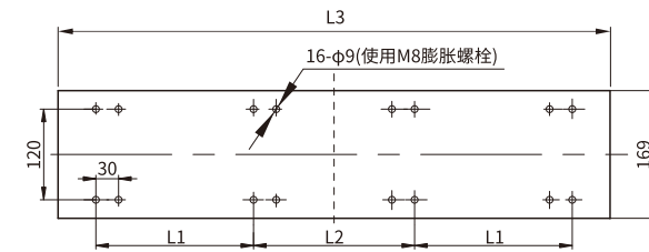
挂墙板尺寸
