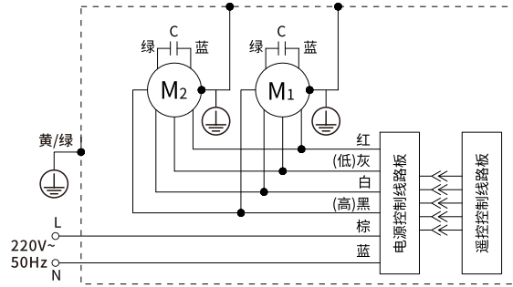
以上原理图适用下列机型 FM3509H-Y-D, FM3512H-Y-D
