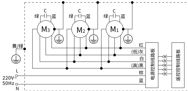
以上原理图适用下列机型 FM3515H-Y-D, FM3518H-Y-D
