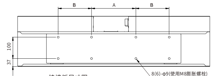
挂墙板尺寸图
