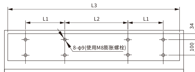
挂墙板尺寸图
