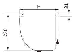
侧面图
